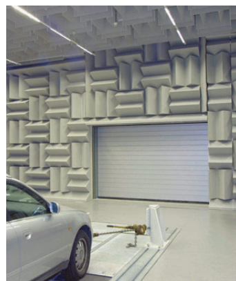
Hubtor geschlossen
