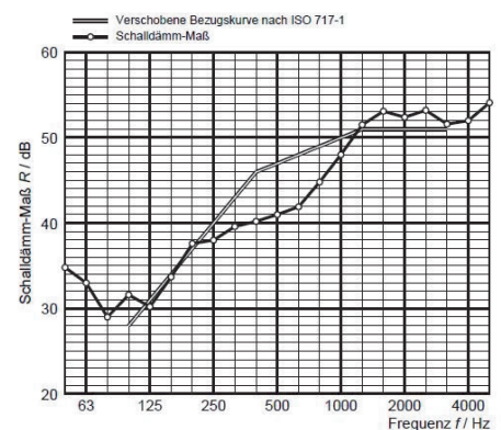
Bewertetes Schalldämm-Maß R_w(C; C_{tr}) = 47 (-2; -5) \text{ dB}
