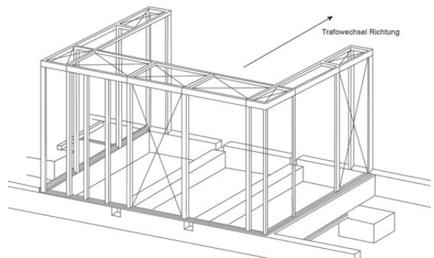
Trafowechsel - Variante 1
