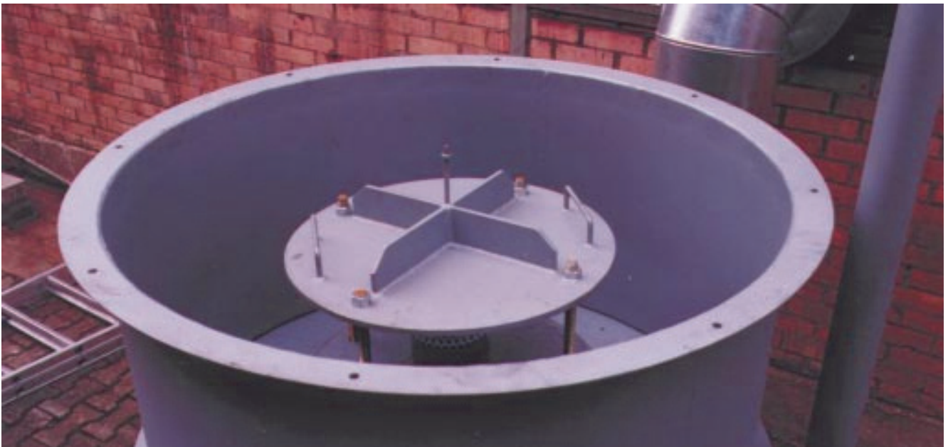
Ausblaseschalldämpfer im Prüfstand
