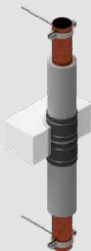
Massivdecke
